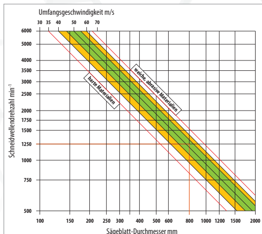
Korrekte Schneidwellendrehzahl Ihrer Maschine in Abhängigkeit von Sägeblattdurchmesser und der Härte des zu schneidenden Materials.
