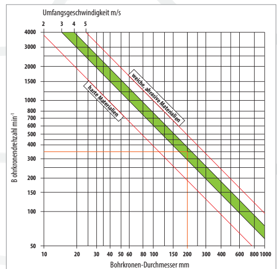
Korrekte Drehzahl Ihres Bohrmotors in Abhängigkeit vom Bohrkronendurchmesser und der Härte des zu bohrenden Materials.
